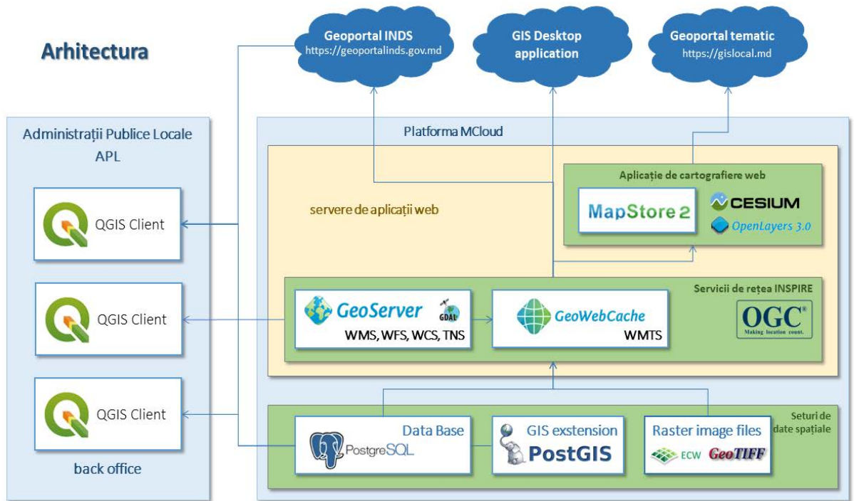
Fig. nr.1. Schema funcțională a SIGSNL și componentele acestuia
