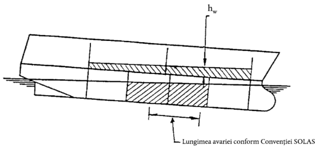
Muchia punții nescufundată
