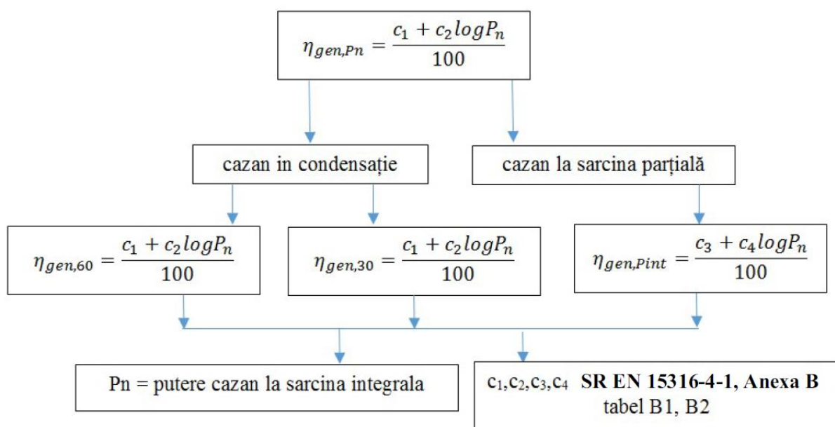
Figura 7.1. Determinarea eficienței energetice a unui cazan
