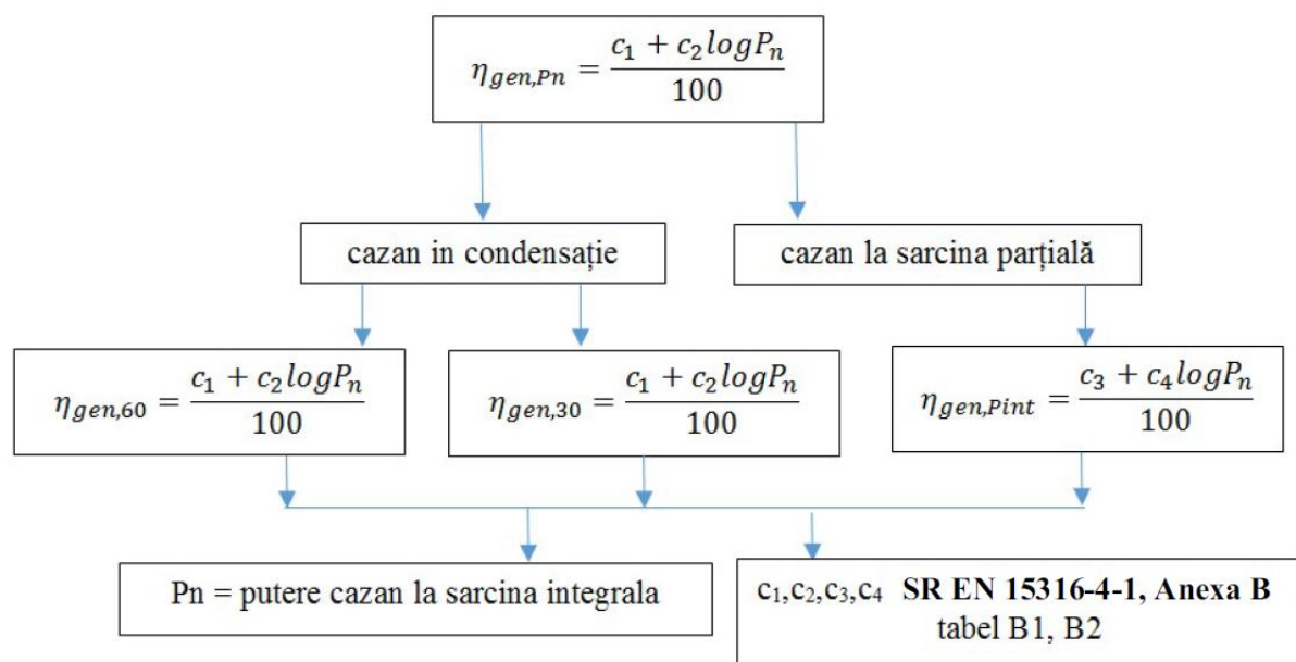
Рисунок 7.1. Определение энергоэффективности котла
