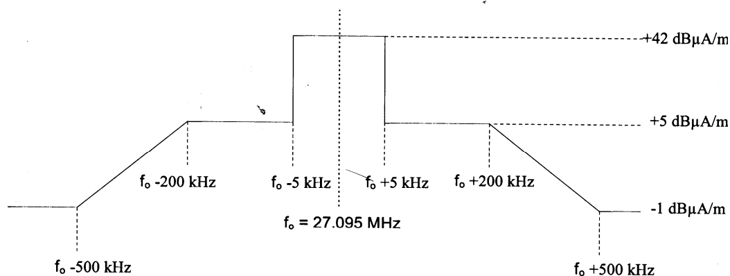
Figura 1: Limitele intensității câmpului magnetic pentru sistemul Eurobaliză la 10 m distanță de măsurare
