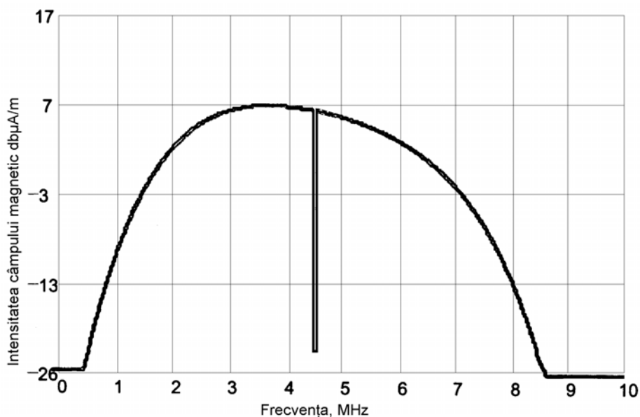
Figura 2: Limitele intensității câmpului magnetic pentru sensul de transmisiune Eurobuclă la Eurobaliză la 10 m distanță de măsurare
